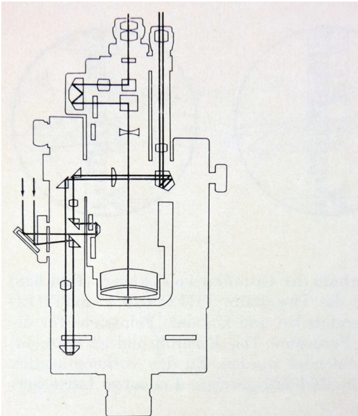
Bild 627. Strahlengang im Dählta 010 Die Kennziffer der Tachymeter des VEB Carl Zeiss JENA gibt den mittleren Ent- fernungsfehler in cm/100 m an
